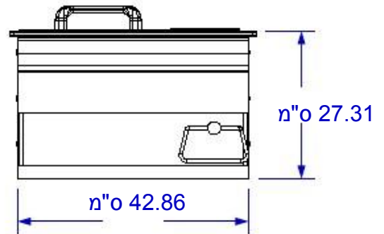
מבט חזיתי
