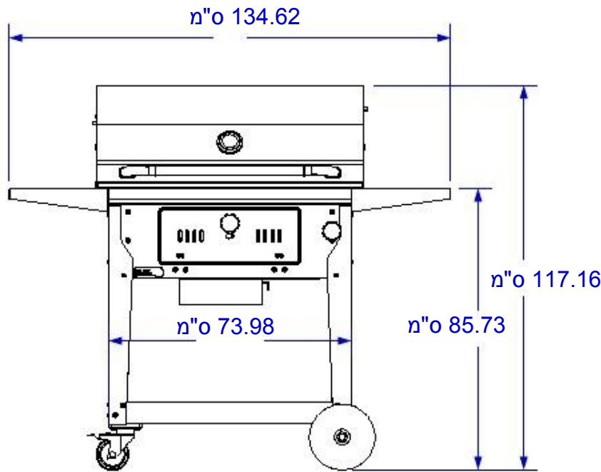
מבט חזיתי
