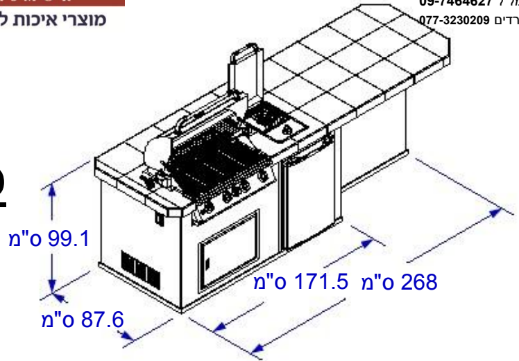
מבט חזיתי איזומטרי
