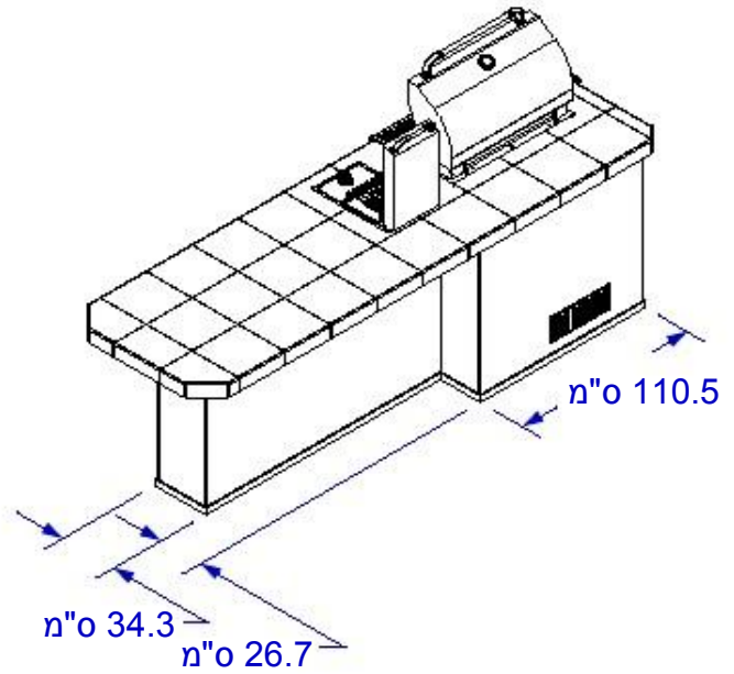
מבט אחורי איזומטרי
