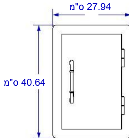
מבט חזיתי
