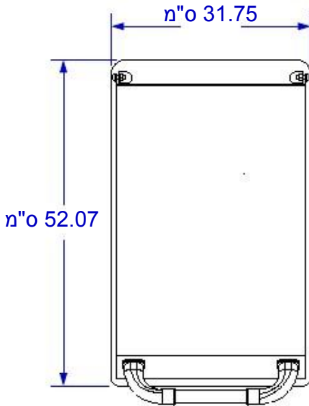
מבט עילי
