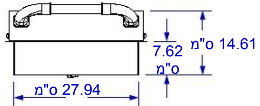
מבט קידמי
