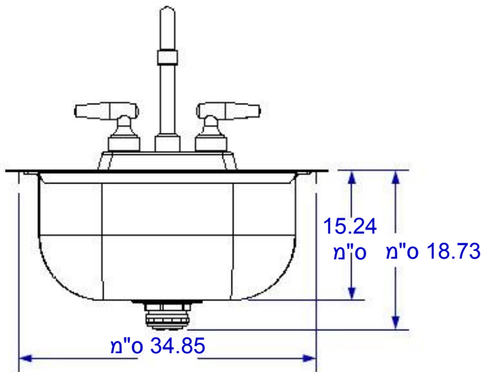
מבט חזיתי
