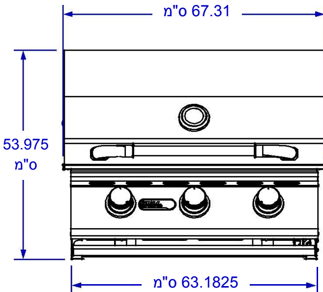
מבט חזיתי
